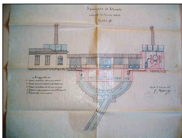
“Stabilimento Balneare di Penne. Progetto d’ingrandimento”, “Spaccato ed elevato secondo la linea ABCD”. Napoli 19 novembre 1886. Disegno a colori su lucido, mm. 458x435, scala 1:100, firmato R. Caputo. [Riproduzione dell’allegato H]. (ARCHIVIO STORICO DEL COMUNE DI PENNE, decennio francese e restaurazione, opere pubbliche , b. 52 n. 37).
