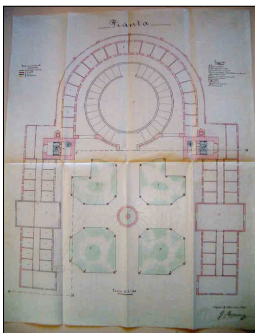
“Stabilimento Balneare di Penne. Progetto d’ingrandimento”, “Pianta”. Napoli 19 novembre 1886. Disegno a colori su lucido, mm. 446x578, scala 1:100, firmato da R. Caputo. [Riproduzione dell’allegato H]. (ARCHIVIO STORICO DEL COMUNE DI PENNE, decennio francese e restaurazione, opere pubbliche , b. 52 n. 37).
