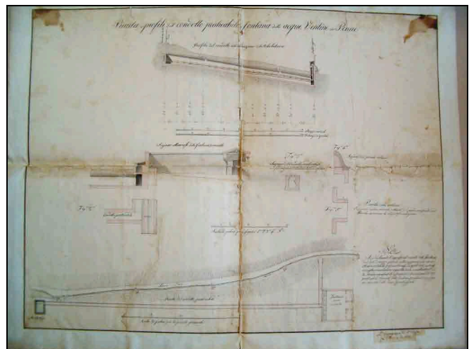
"Pianta e profili del condotto praticabile e fontana delle acque Ventine in Penne". [sec. XIX]. Disegno a colori su carta, mm. 592x473, firmato dall'ingegnere di terza classe Lodovico De Vito. [Riproduzione dell'allegato F]. (ARCHIVIO STORICO DEL COMUNE DI PENNE, decennio francese e restaurazione, opere pubbliche , b. 52 n. 37).
